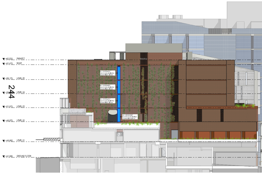
1 E7 ELEVATION_RADNOR 1:150
